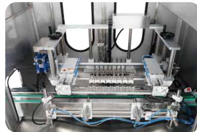
洗瓶机内部图
